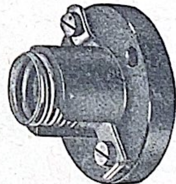
Isolierstoff-Fassung E 10 (1548)
