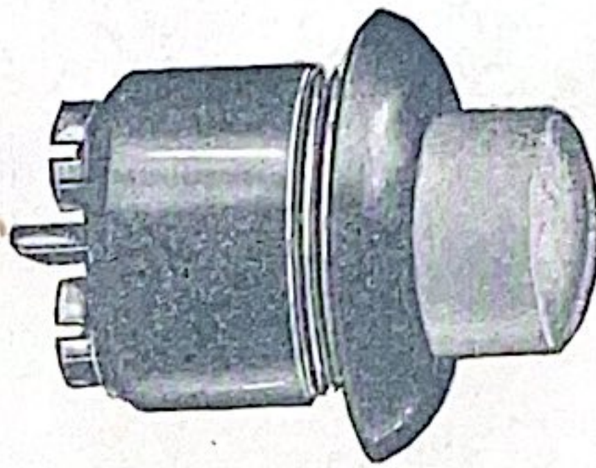
Einschraubkontakt Nr. 100 A und 101 A (1243) (1244)
