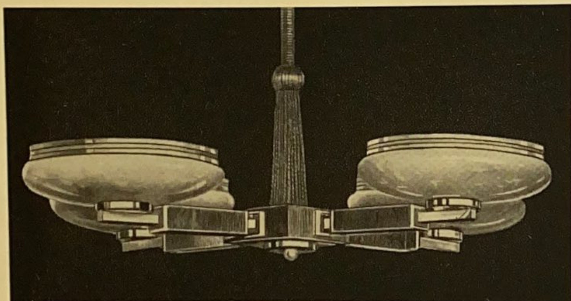
Ld 304 4 Lp. D 72 cm L 90 cm 4 Gläser Nr. 020/22 cm Holz, Metallteile veredelt Güteklasse 1
