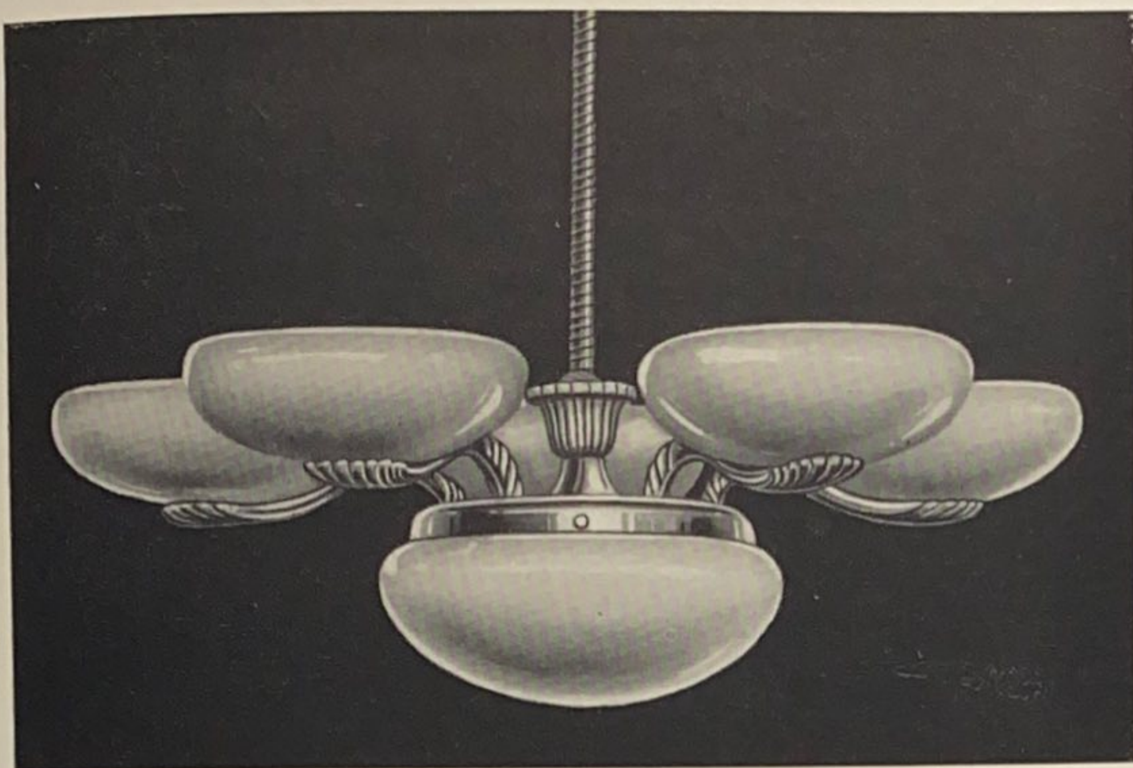
Ld 318 5+1 Lp. D-66 cm L 100 cm 1 Unterglas Nr. 024/26 × 20 cm 5 Gläser Nr. 01/21 cm Gußteile veredelt Güteklasse 2
