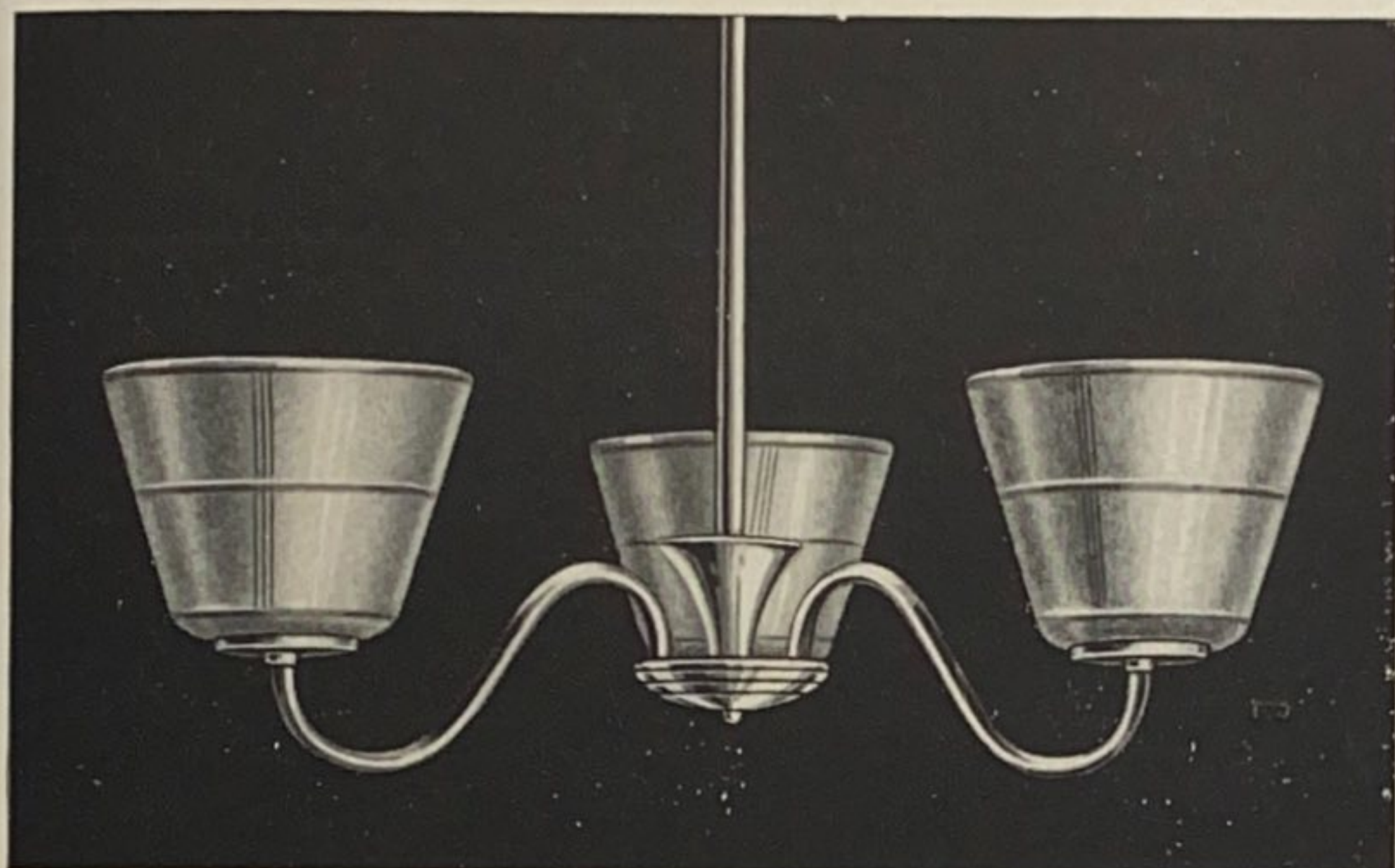
A 682 3 Lp. D 55 cm L 90 cm 3 Gläser 2602/7593 transparent 17 cm Metall messingfarbig
