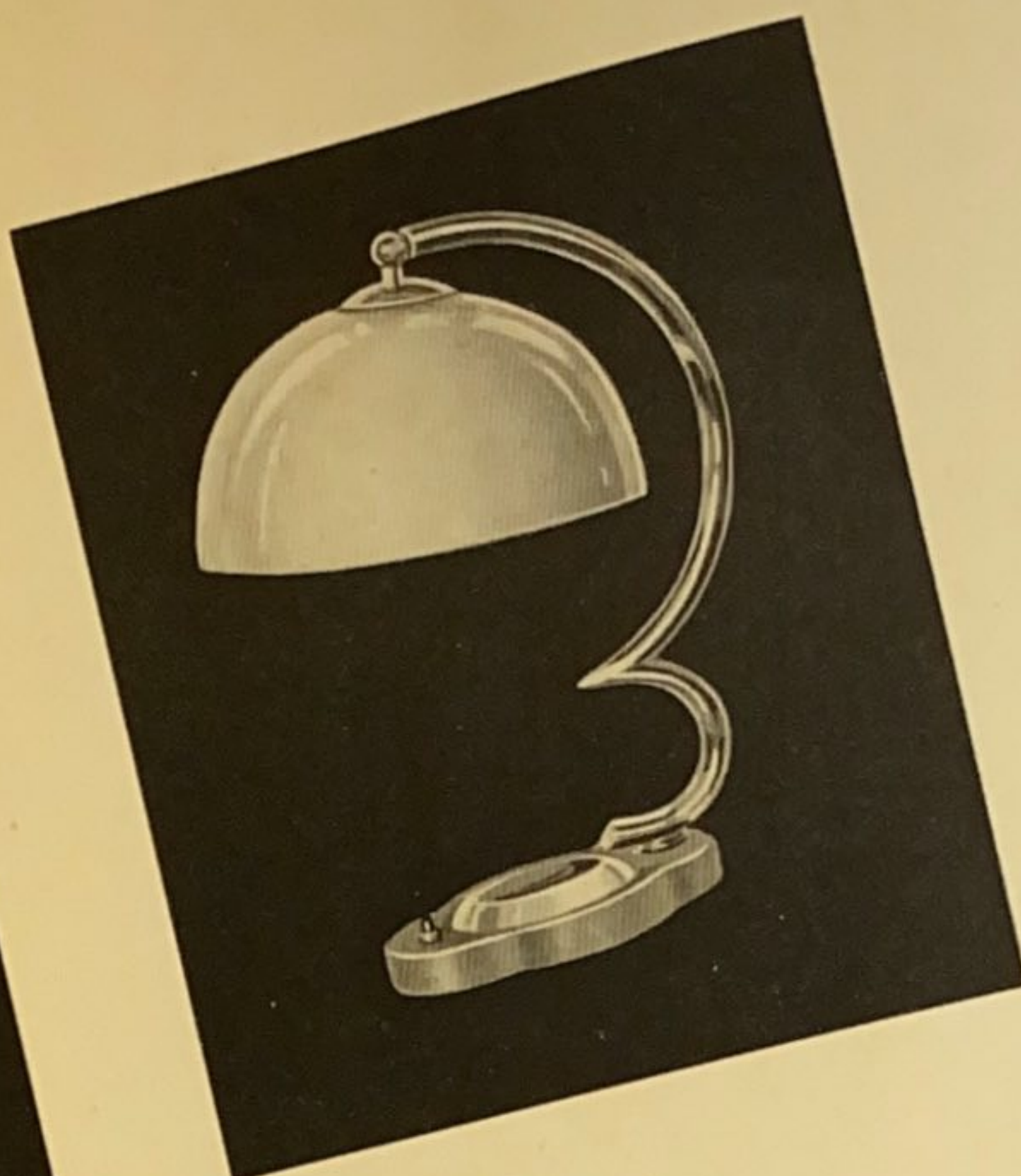
Ld 812 1 Lp. H 40 cm 1 Glas Nr. 042/26 cm Serpentinsteine, Metallteile veredelt Gütekategorie 2
