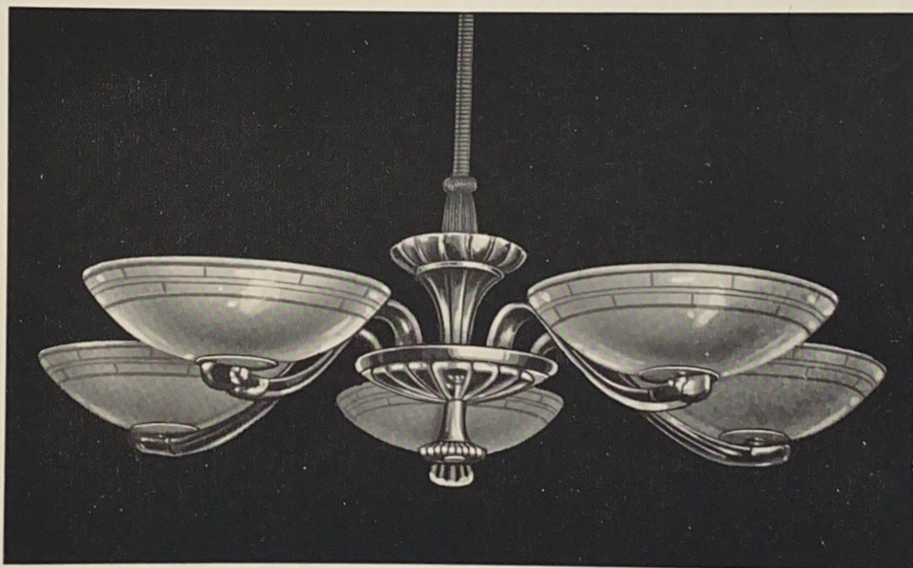
A 686 5 Lp. D 95 cm L 100 cm 5 Gläser 2854/280 transp. mit Dekor Guß messingfarbig
