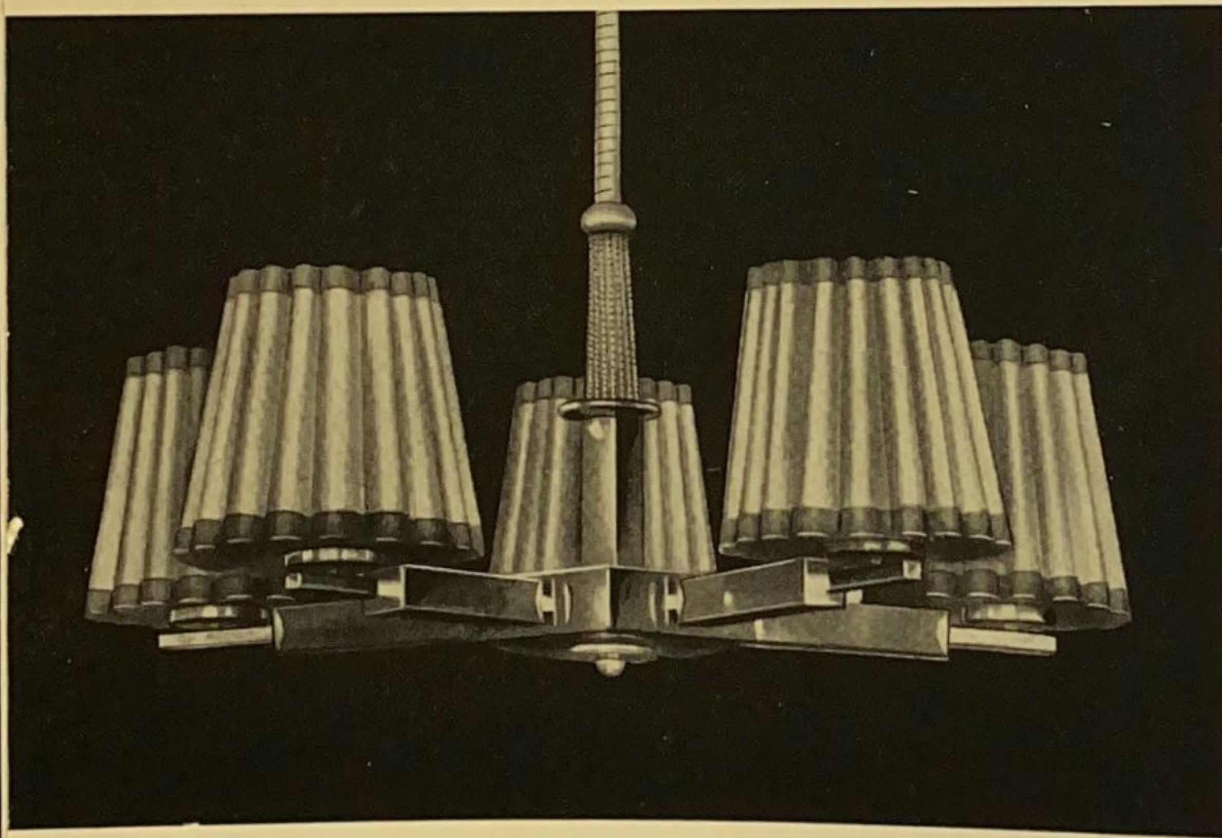
Ld 404a 5 Lp. D 66 cm L 100 cm 5 Schirmchen Nr. 016/16 cm Holz, Metallteile veredelt Güteklasse 1
