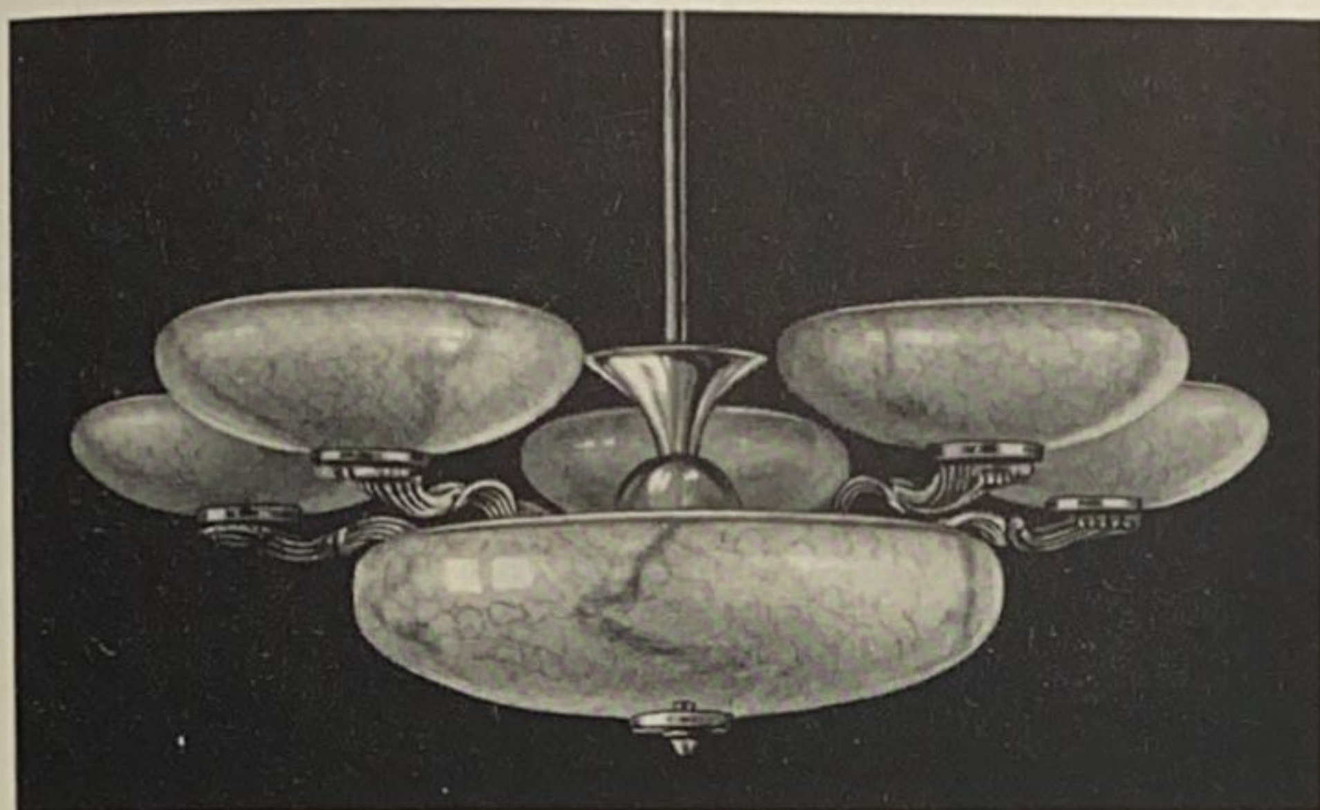
A 665 5+2 Lp. D 75 cm L 100 cm 1 Unterglas 2747/40 cm champ. marm. 5 Gläser 1263/23 cm champ. marm. Guß messingfarbig
