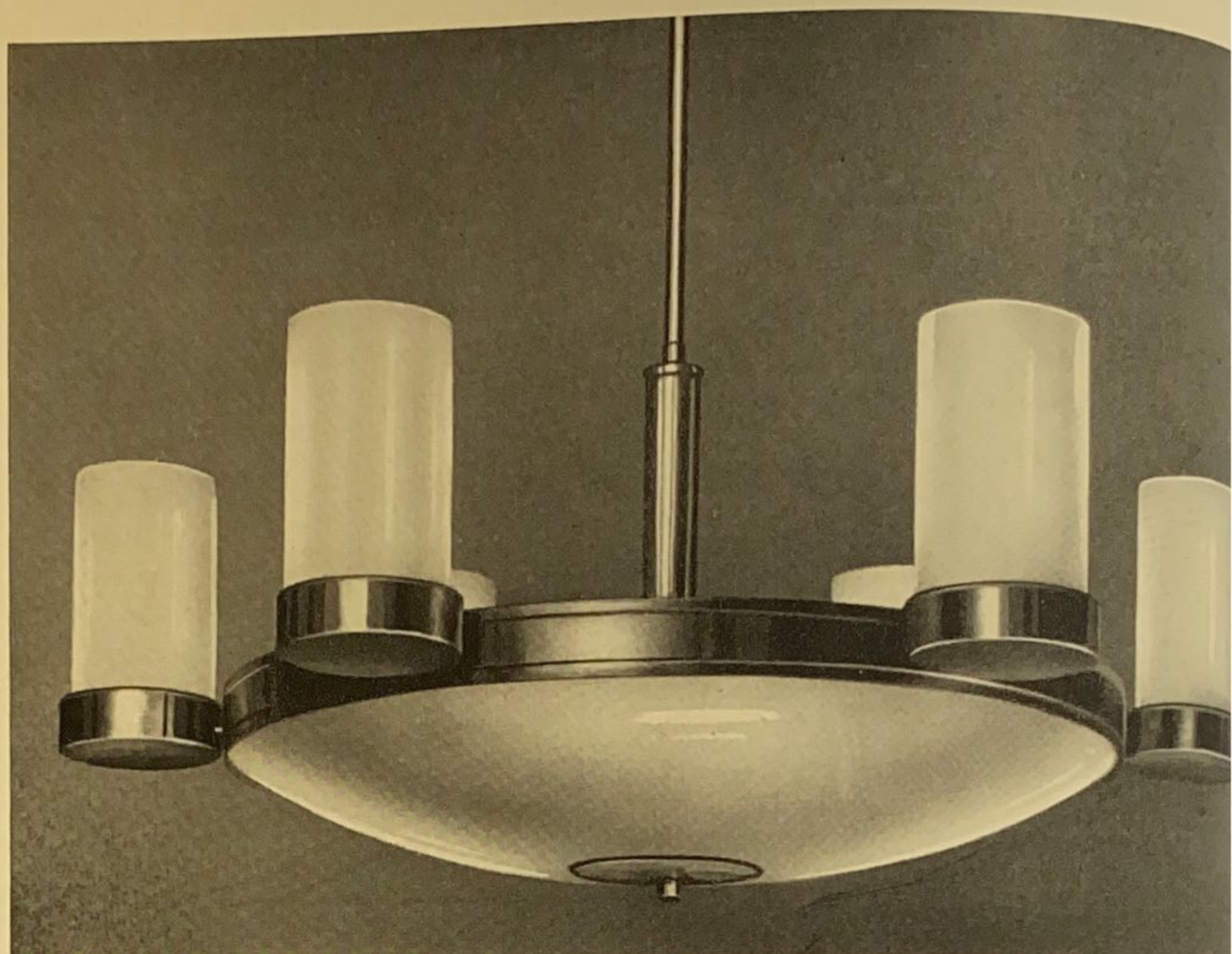
D 40808 6+3 Lp. D 90 cm L 110 cm 1 Unterglas 10111 damp. 6 Gläser 10152 damp. Metall messingfarbig
