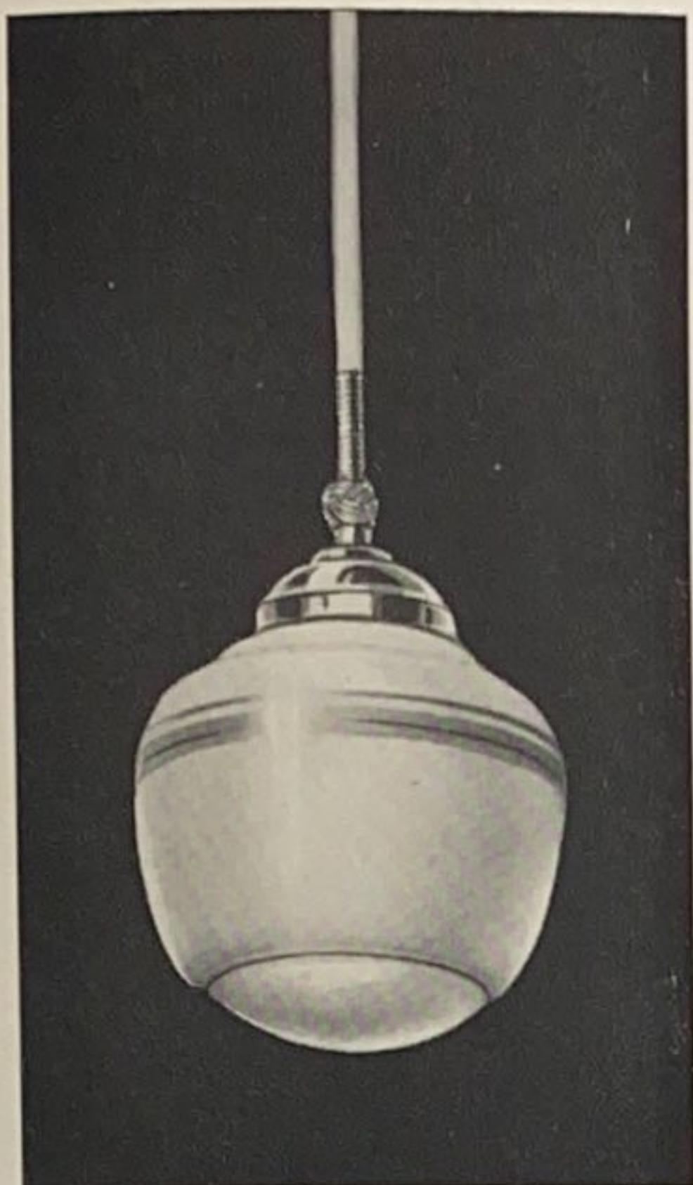
Ld 1180 1 Lp. m. 80er Halter D 18 cm L 75 cm 1 Glas Nr. 044/18 cm Lackiert Güteklasse 2
