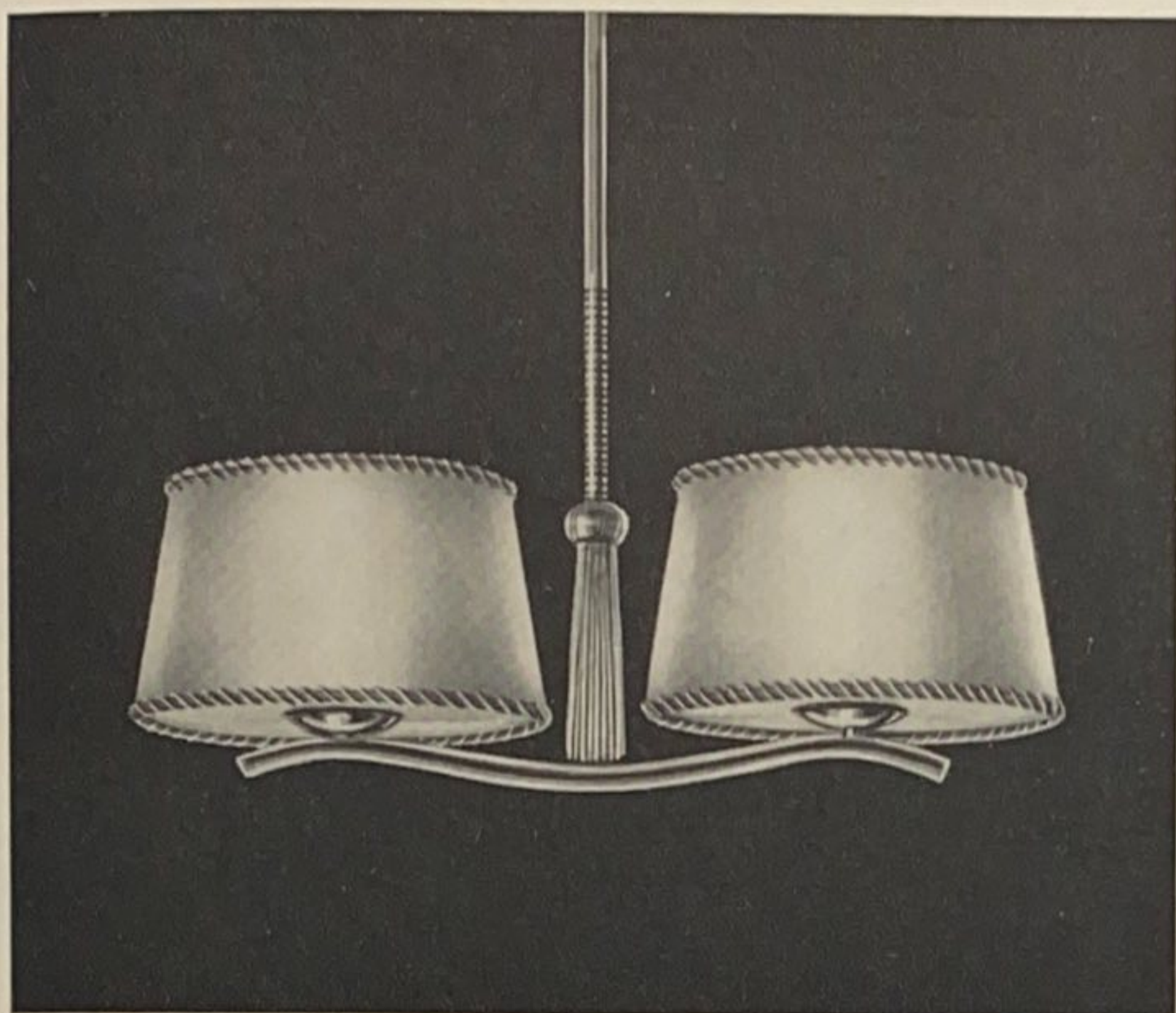
Ld 104 2 Lp. D 50 cm L 90 cm 2 Schirmchen Nr. 015/22 cm mit 2 Glasplatten Mattglas Metallteile veredelt Güteklasse 1
