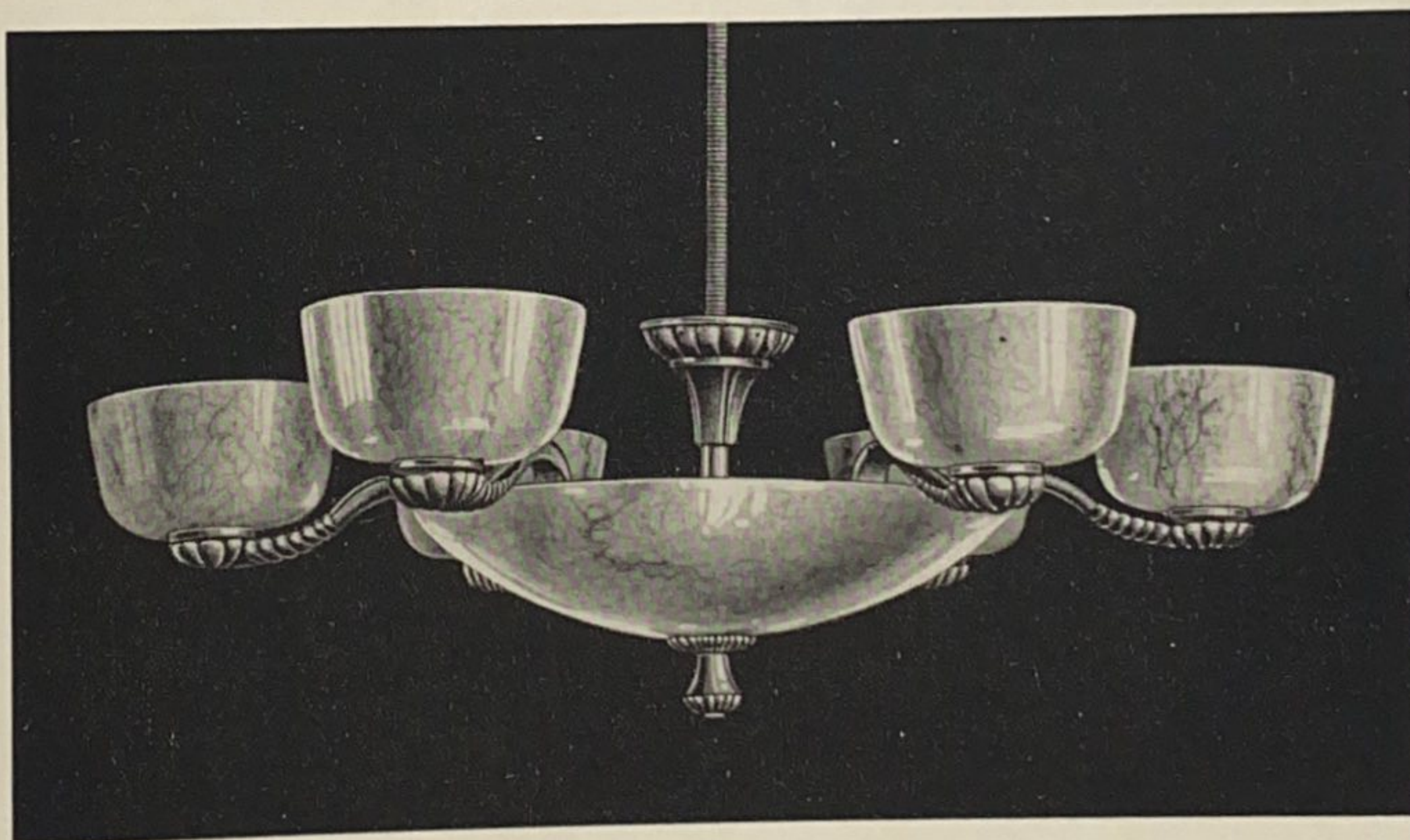
A 680 6+3 Lp. D 105 cm L 100 cm 1 Unterglas 48 cm champ. marm. 6 Gläser 2615/20 cm champ. marm. Guß messingfarbig
