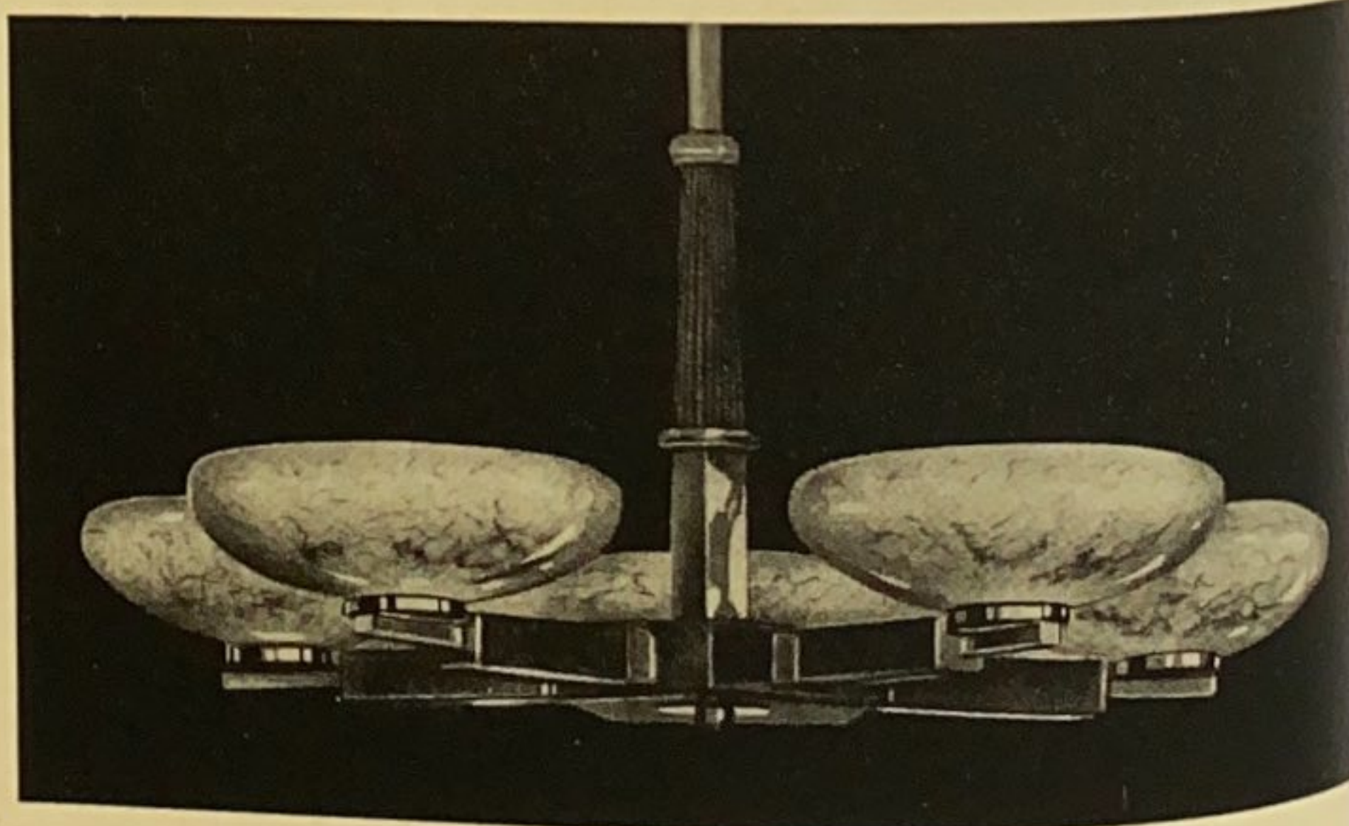
Ld 404 5 Lp. D 72 cm L 100 cm 5 Gläser Nr. 07/22 cm Holz, Metallteile veredelt Güteklasse 1
